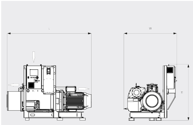
尺寸圖
