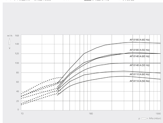
抽氣速率
