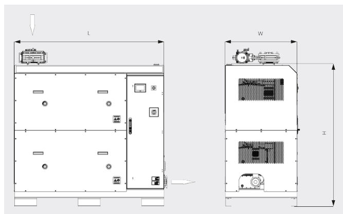
尺寸圖
