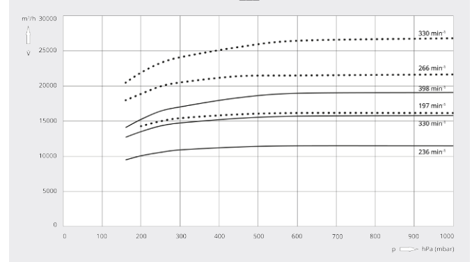
抽氣速率
