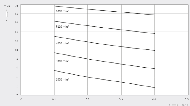
抽氣速率
