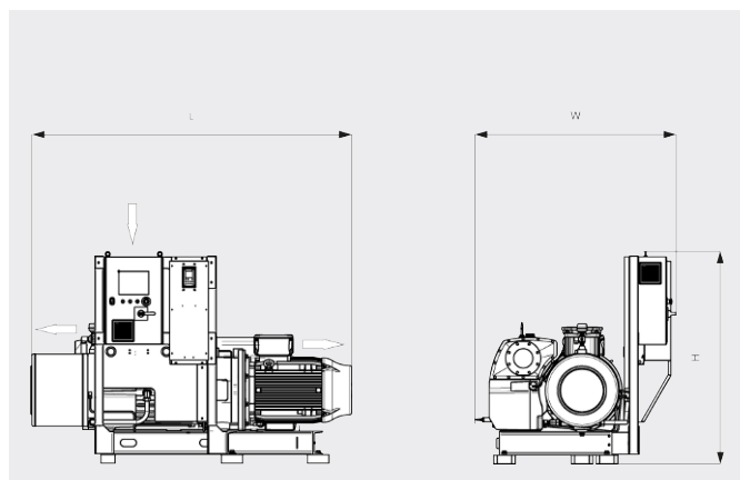
尺寸圖
