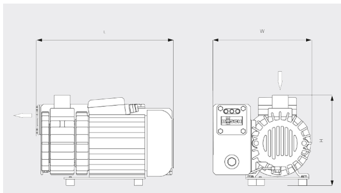
尺寸圖
