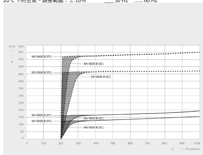
抽氣速率
