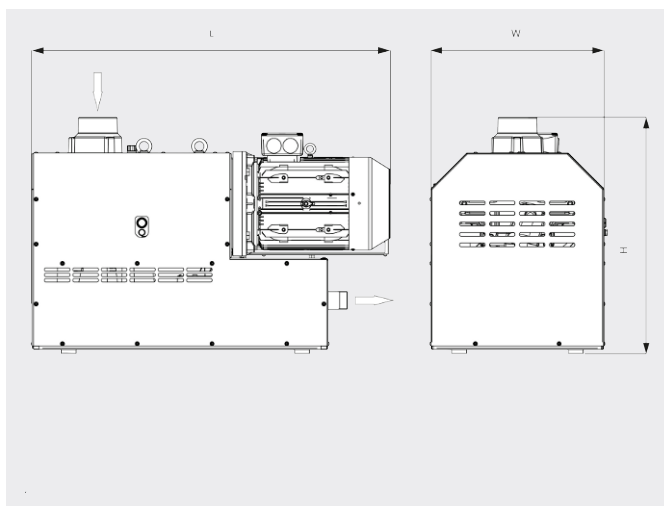
尺寸圖
