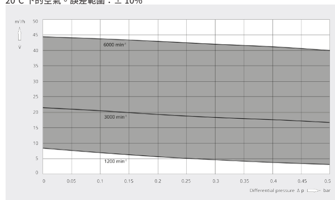
體積流量（進氣口） 20°C 下的空氣。誤差範圍：± 10%
