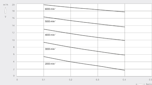
抽氣速率
