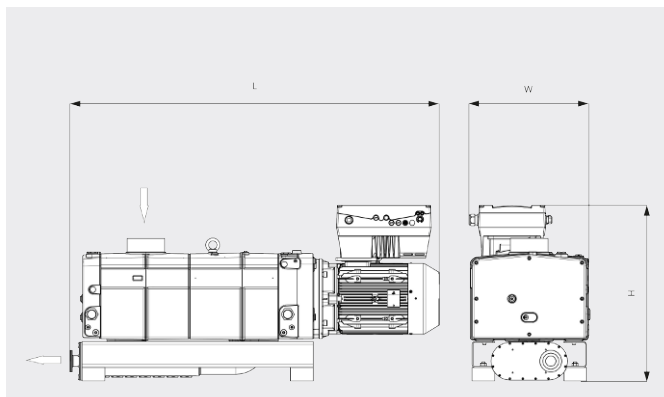
Måttitritning
