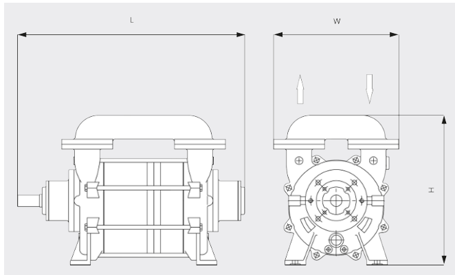
Måttritning
