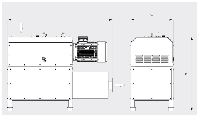
Måttritning
