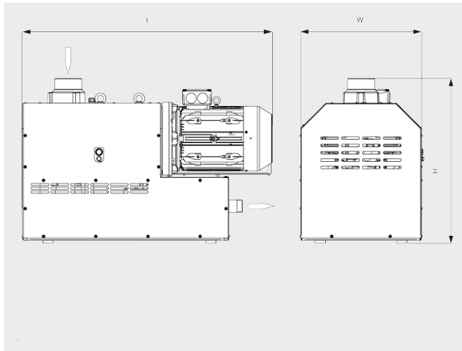
Måttritning
