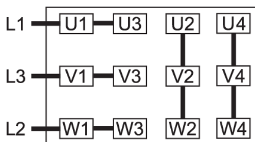
Stjärnkoppling, flerspänningsmotor med 12 stift (hög spänning):
