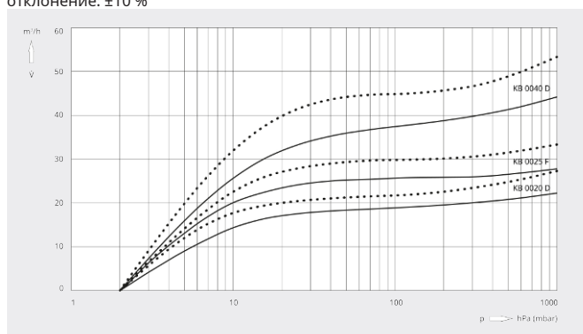
Скорость откачки Воздух при 20 °С. Допустимое отклонение: ±10 %
