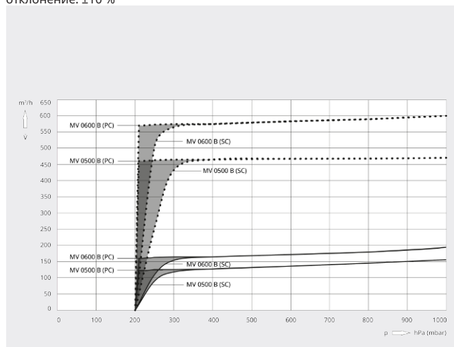
Скорость откачки Воздух при 20 °С. Допустимое отклонение: ±10 %
