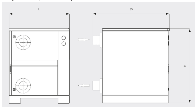
Габаритный чертеж (с шумоизоляционным кожухом)
