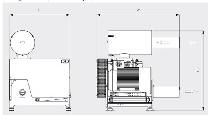
Габаритный чертеж (без шумоизоляционного кожуха)
