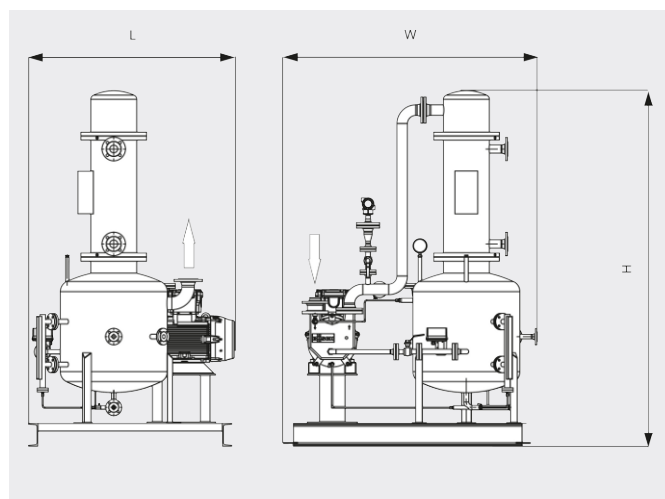
Desen dimensional
