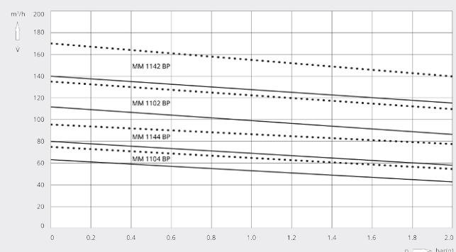
Wydajność pompowania
