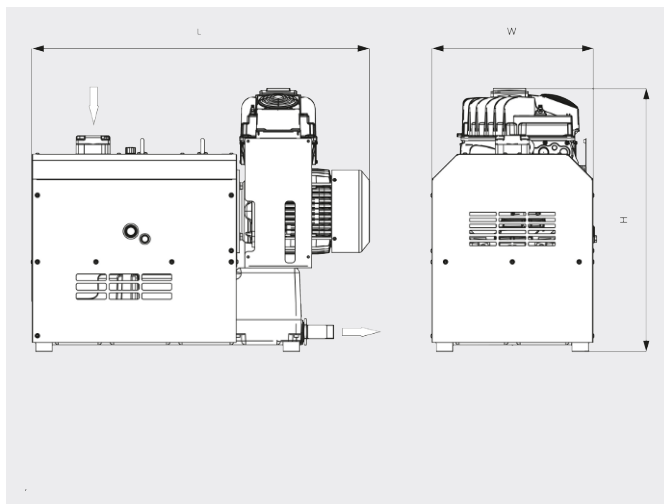
Dibujo dimensional
