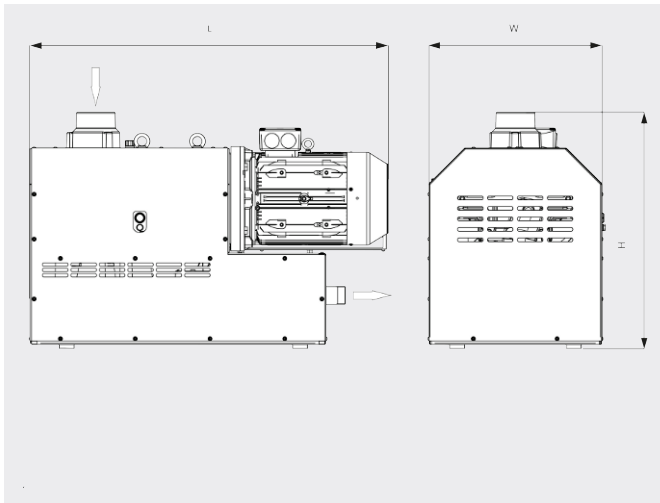
Målskisse
