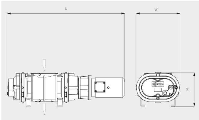
Dimensjonstegning
