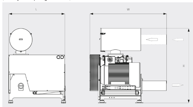
Dimensjonstegning (uten lyddempningskabinett)
