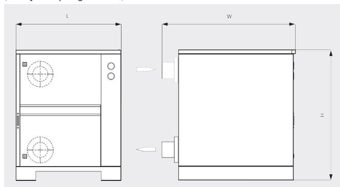
Dimensjonstegning (med lyddempningskabinett)
