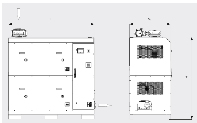
Dimensjonstegning
