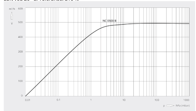
Pumpekapasitet Luft ved 20 °C. Toleranse: ±10 %
