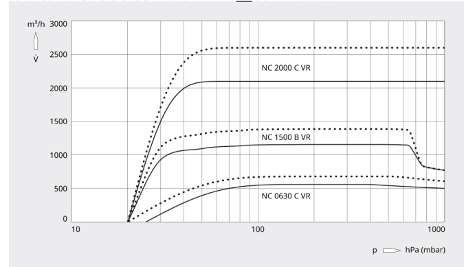
Pumpekapasitet
