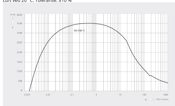
Pumpekapasitet
