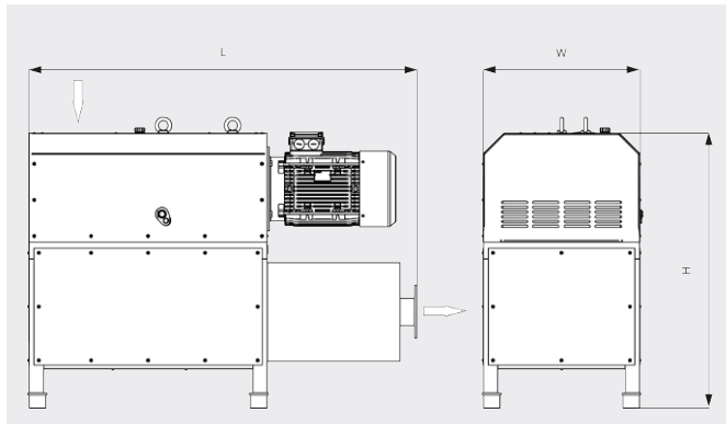
Målskisse
