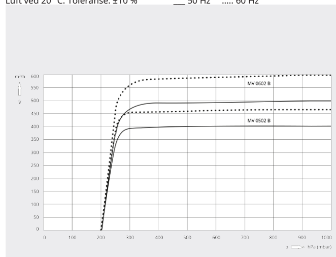
Pumpekapasitet
