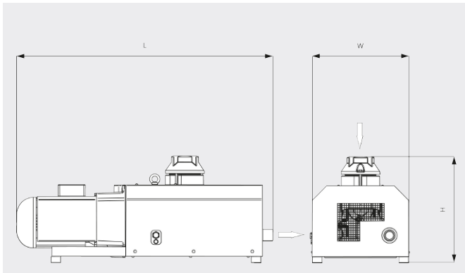
Målskisse
