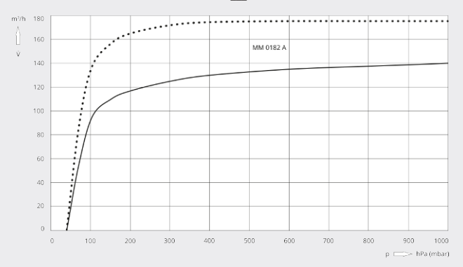
Pumpekapasitet
