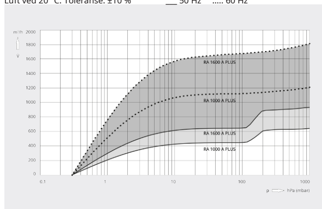
Pumpekapasitet
