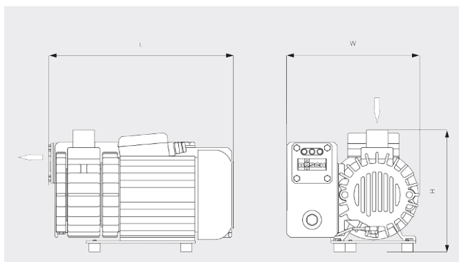
Dimensjonstegning
