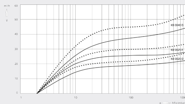
Pumpekapasitet
