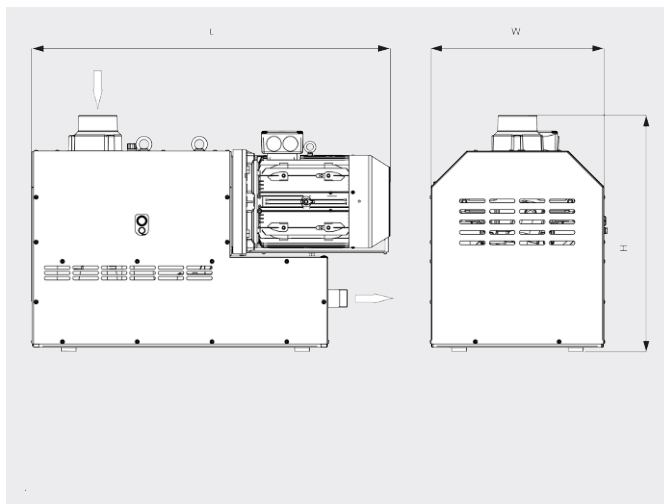
Målskisse
