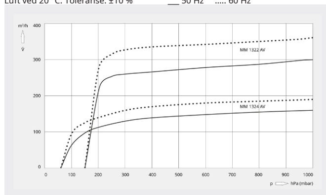
Pumpekapasitet
