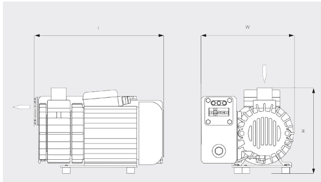
Dibujo dimensional
