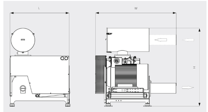
치수 도면 (방음 케이스 미포함)
