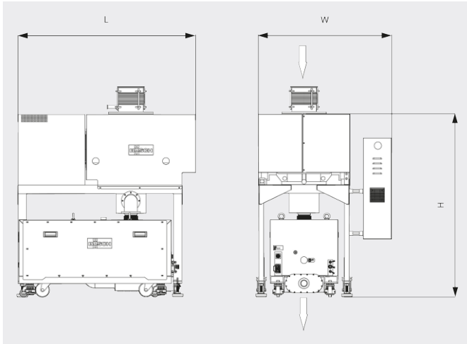
치수 도면
