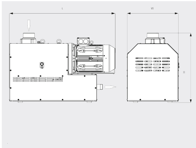
치수 도면
