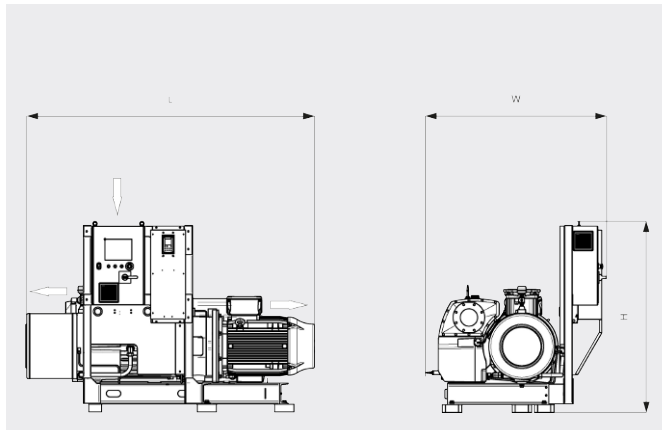
치수 도면
