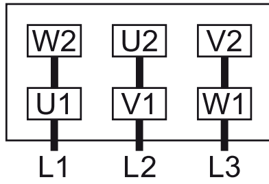
デルタ接続（低電圧）：
