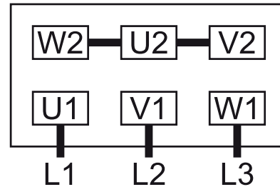
スター接続（高電圧）：
