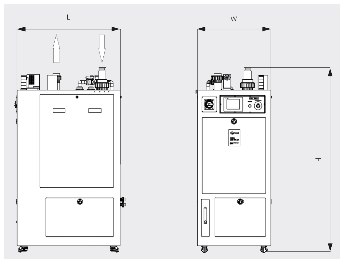
寸法図
