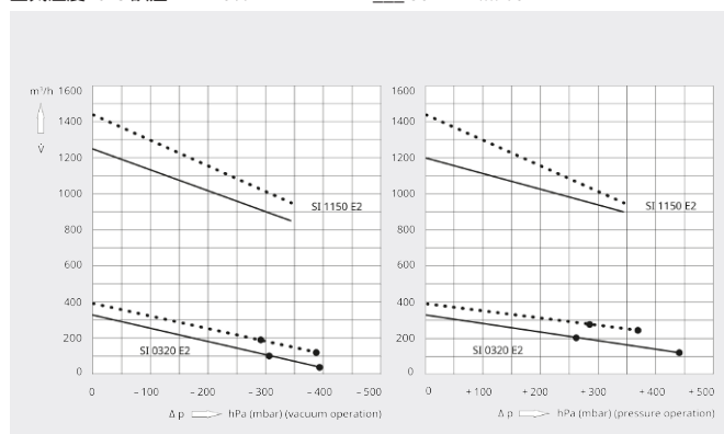
排気速度/排気量 空気温度20°C 誤差: ± 10%
