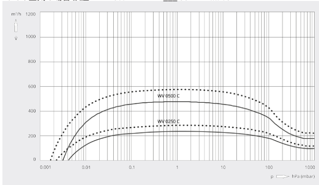
排気速度
