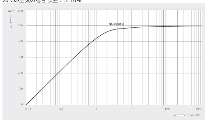
排気速度 20°Cの空気の場合 誤差：± 10%
