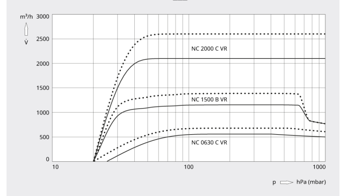
排気速度
