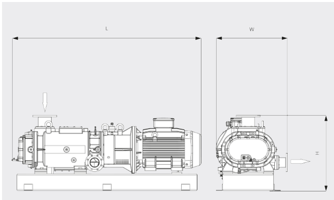
外形寸法図
