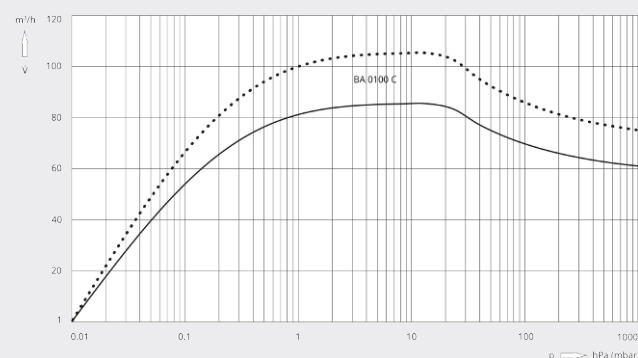
排気速度
