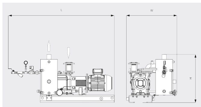
寸法図 (安全区域)
