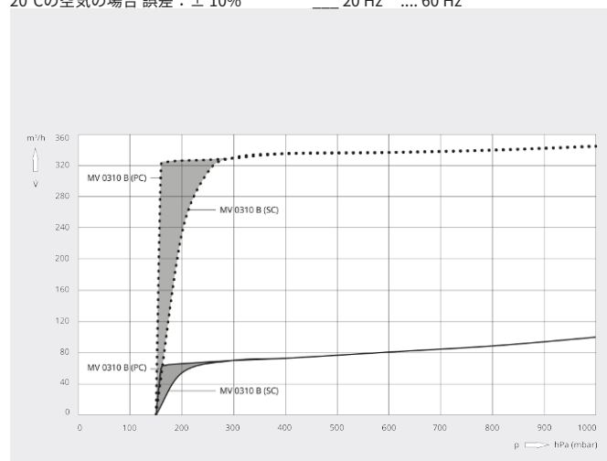
排気速度
